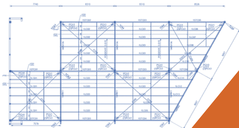
PLANTA DE CUBIERTA
